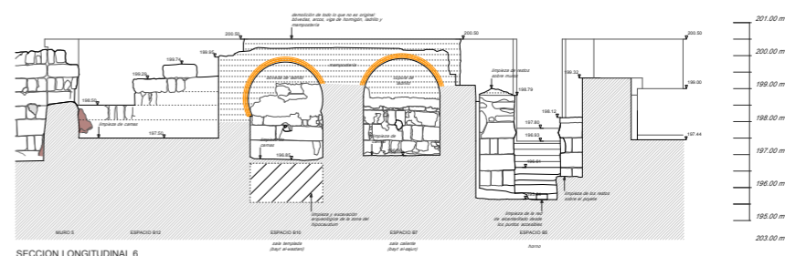
SECCION LONGITUDINAL 6
