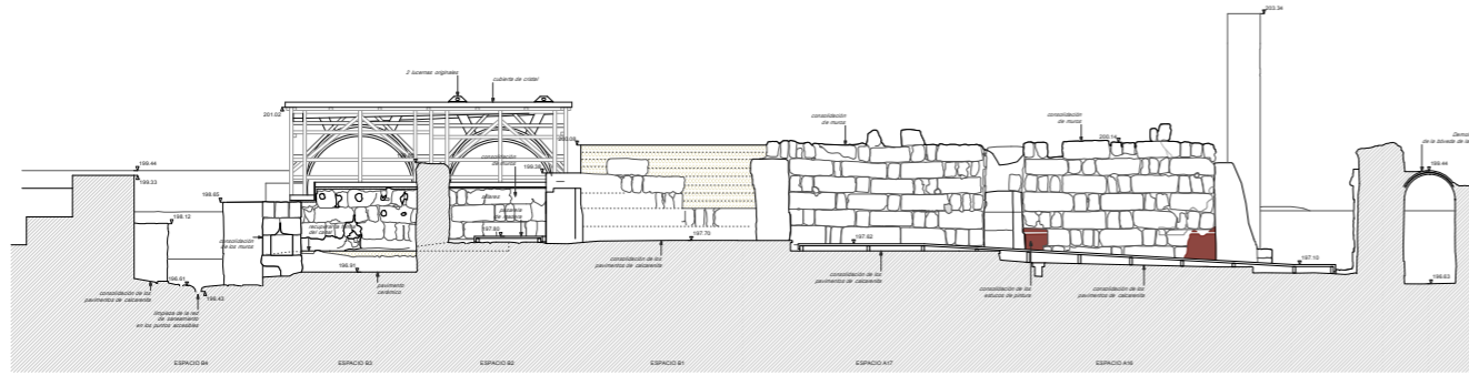
SECCIÓN LONGITUDINAL 10
