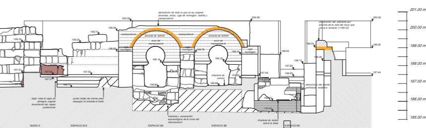
SECCION LONGITUDINAL 4
