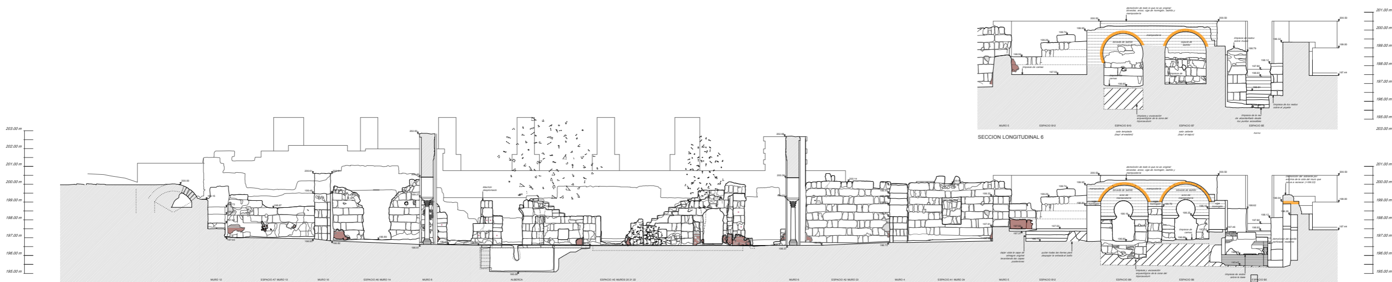
SECCION LONGITUDINAL 5
