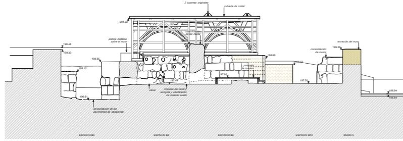
SECCIÓN LONGITUDINAL 11
