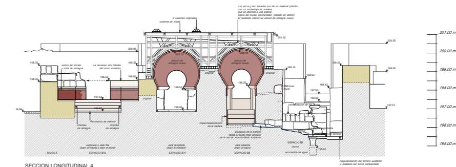
SECCION LONGITUDINAL 4
