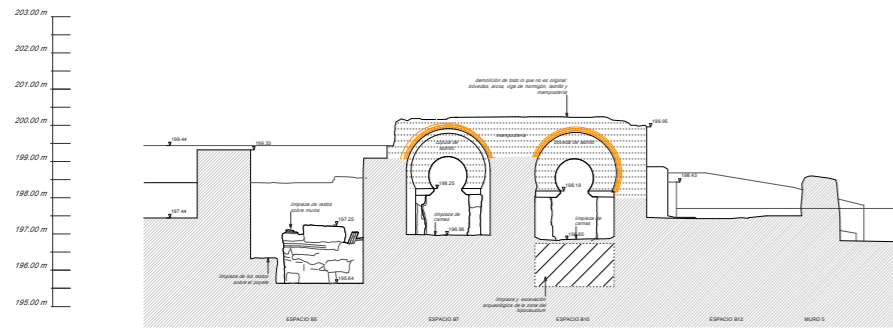
SECCION LONGITUDINAL 12
