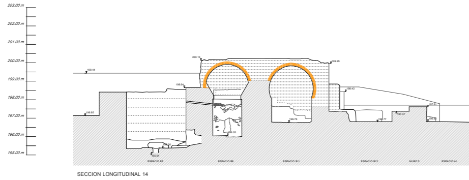
SECCION LONGITUDINAL 14
